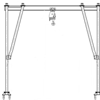
Рис. 2 Конструкция с раскосами (более устойчивая)
