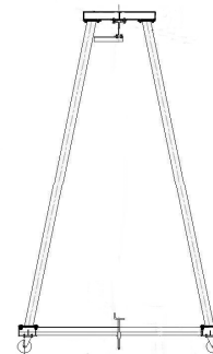
Рис. 2 Конструкция с раскосами (более устойчивая)
